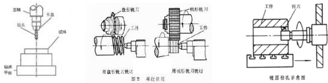
铣床的加工范围
