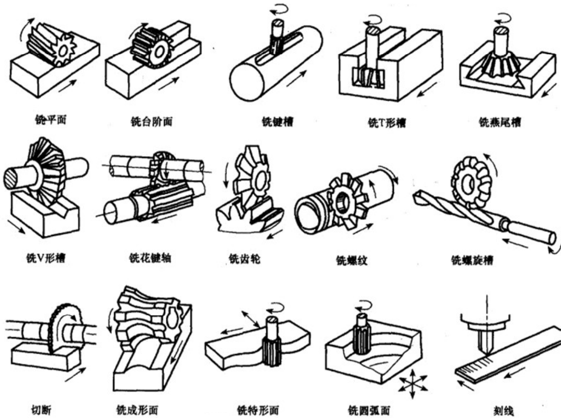
铣床的加工范围
