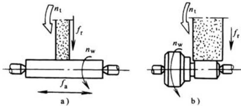
外圆磨床的磨削方法
