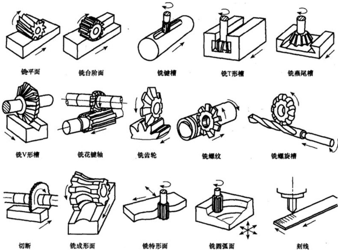
铣床的加工范围
